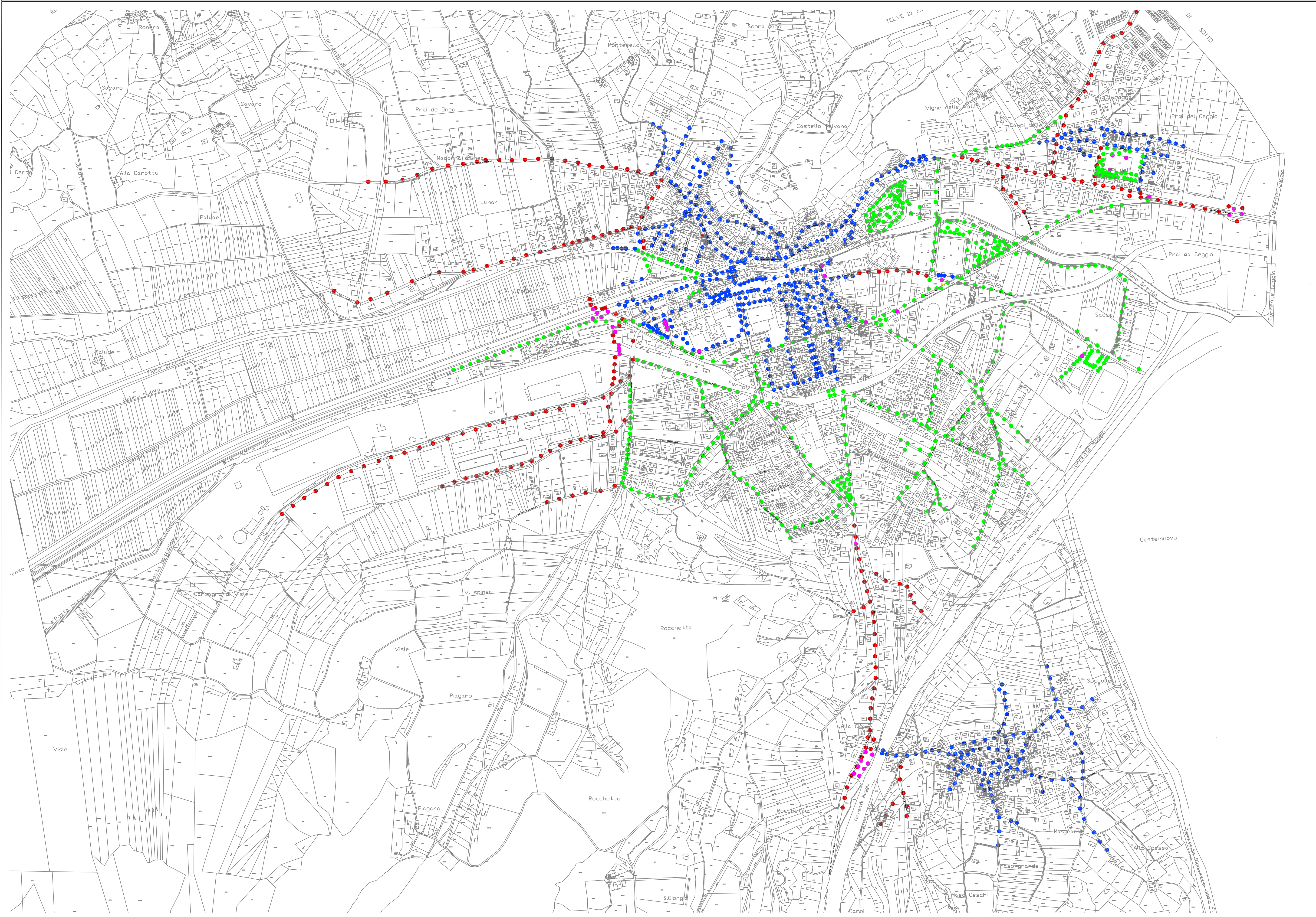
TAVOLA STATISTICA APPARECCHI SELLA (scala 1:5000)
